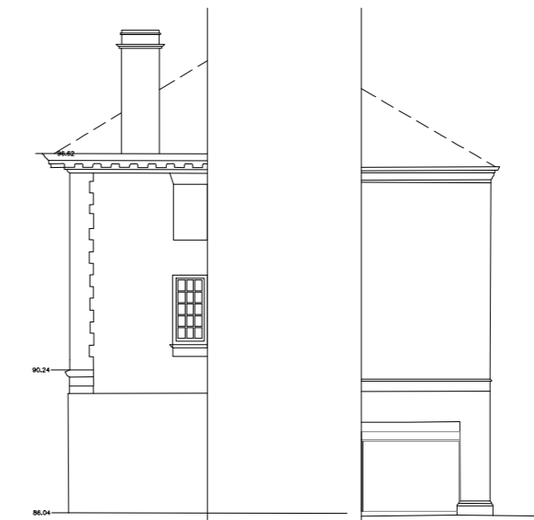
Existing elevation 5
